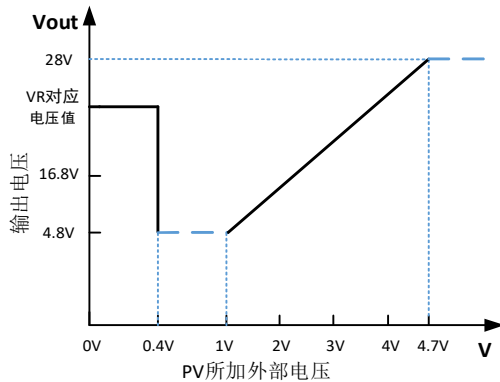
负载曲线
