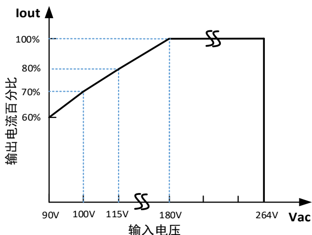
GW-1800W-12V/24V/48V 输出降额曲线
