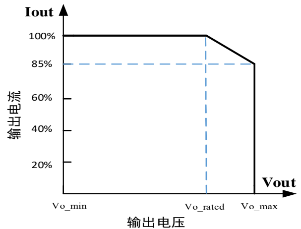
负载曲线
