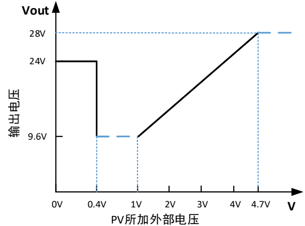
GW-1800W-24 主路输出 PV 调压曲线
