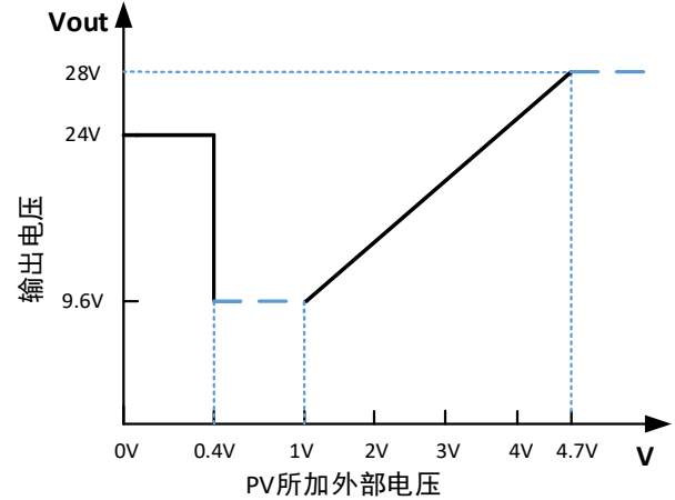
GW-1100W-24 主路输出 PV 调压曲线
