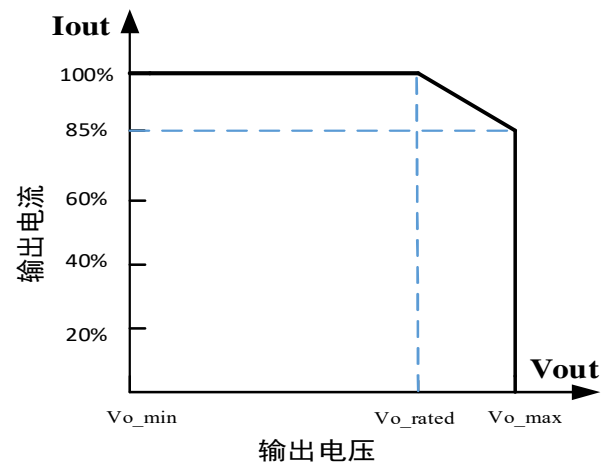
负载曲线
