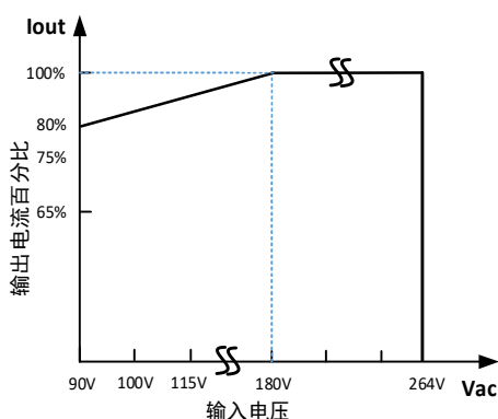
GW-2200W-12V 输出降额曲线
