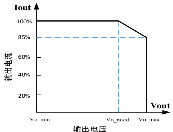
负载曲线
